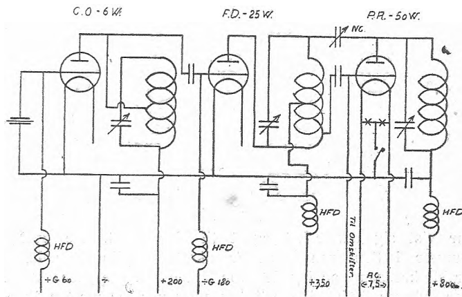
Senderdiagram.
